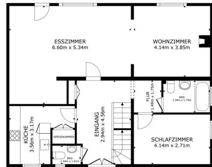
STOCKWERK 2
