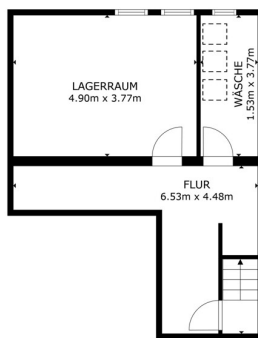
STOCKWERK 1
